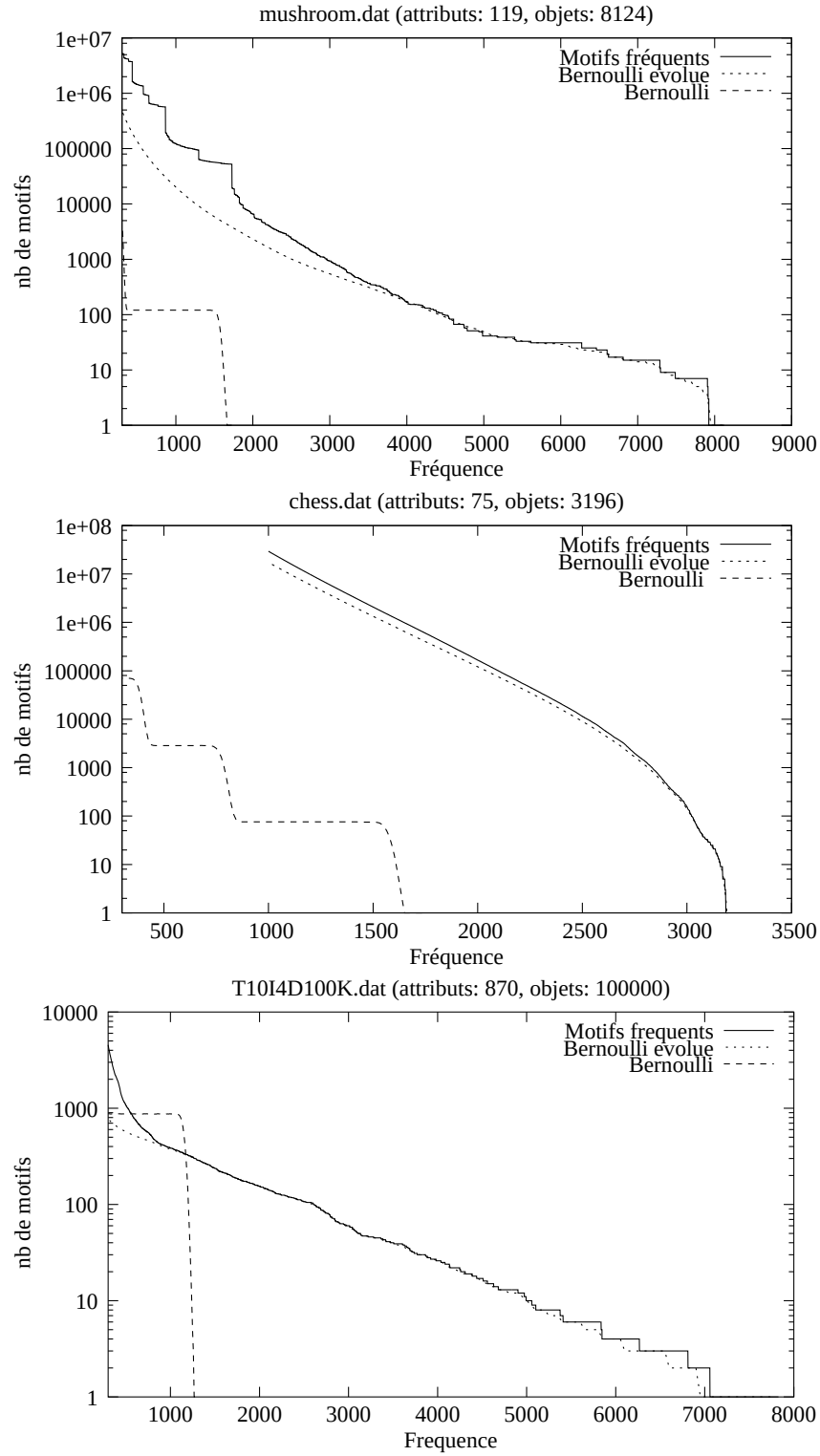
FIG. 7.5 – Comparaison entre le nombre de motifs fréquents présents réellement, le nombre de motifs fréquents théoriques issu de modèle de Bernoulli et le nombre de motifs fréquents théoriques issu de modèle de Bernoulli évolué.
