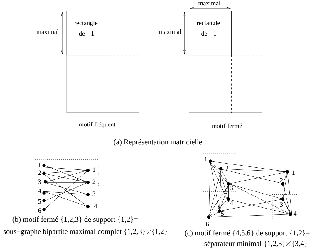
FIG. 6.10 – Correspondances entre les motifs fréquents ou fermés et les rectangles maximaux dans la matrice, les sous-graphes bipartites complets maximaux et les séparateurs minimaux.
