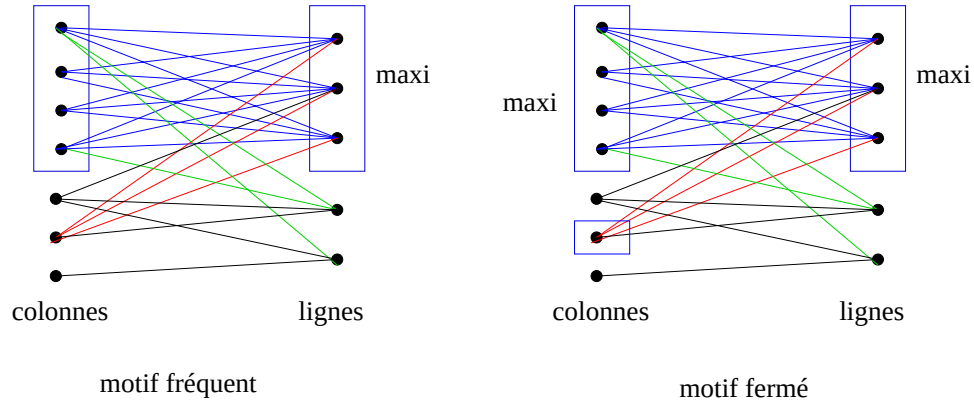
FIG. 7.3 – Liens entre les motifs fréquents ou fermés avec les sous-graphes bipartites complets.
