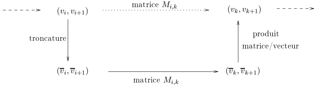
FIG. 1.2 – Une étape de l’algorithme de Lehmer-Euclide.
